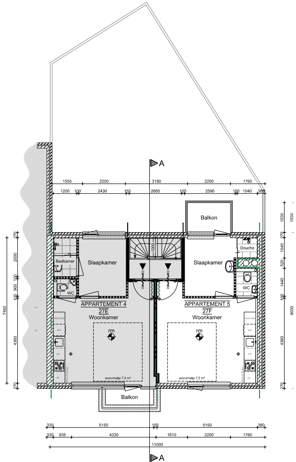
3e Verdieping - NIEUW 9375+P
