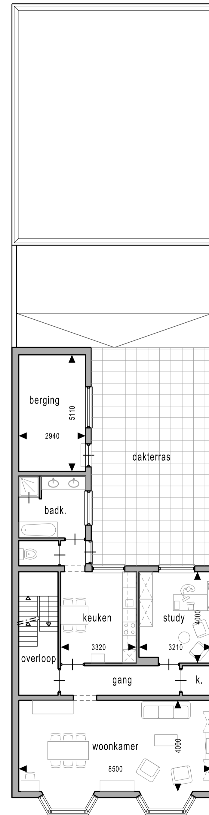
1e VERDIEPING
