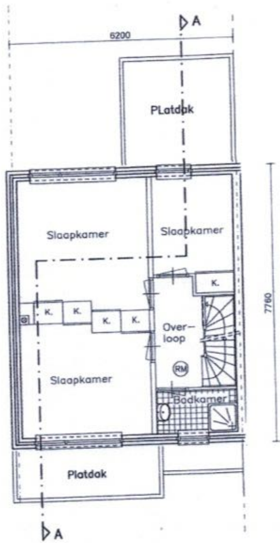
Eerste verdieping
