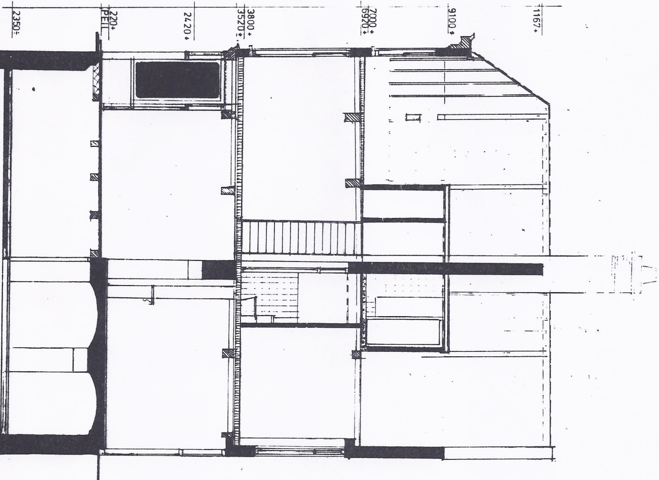
doorsnede A-A
