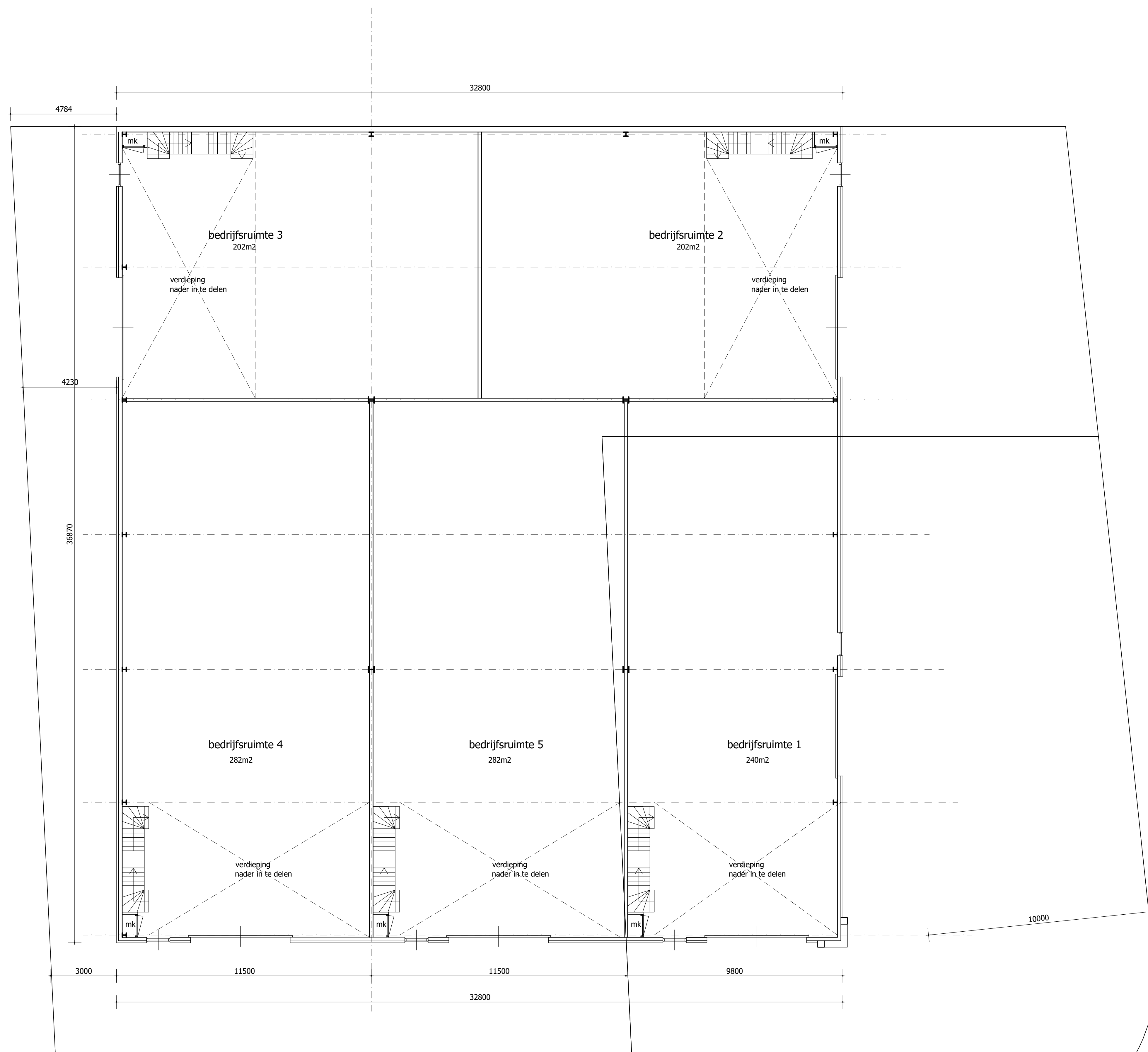
BEGANE GROND
