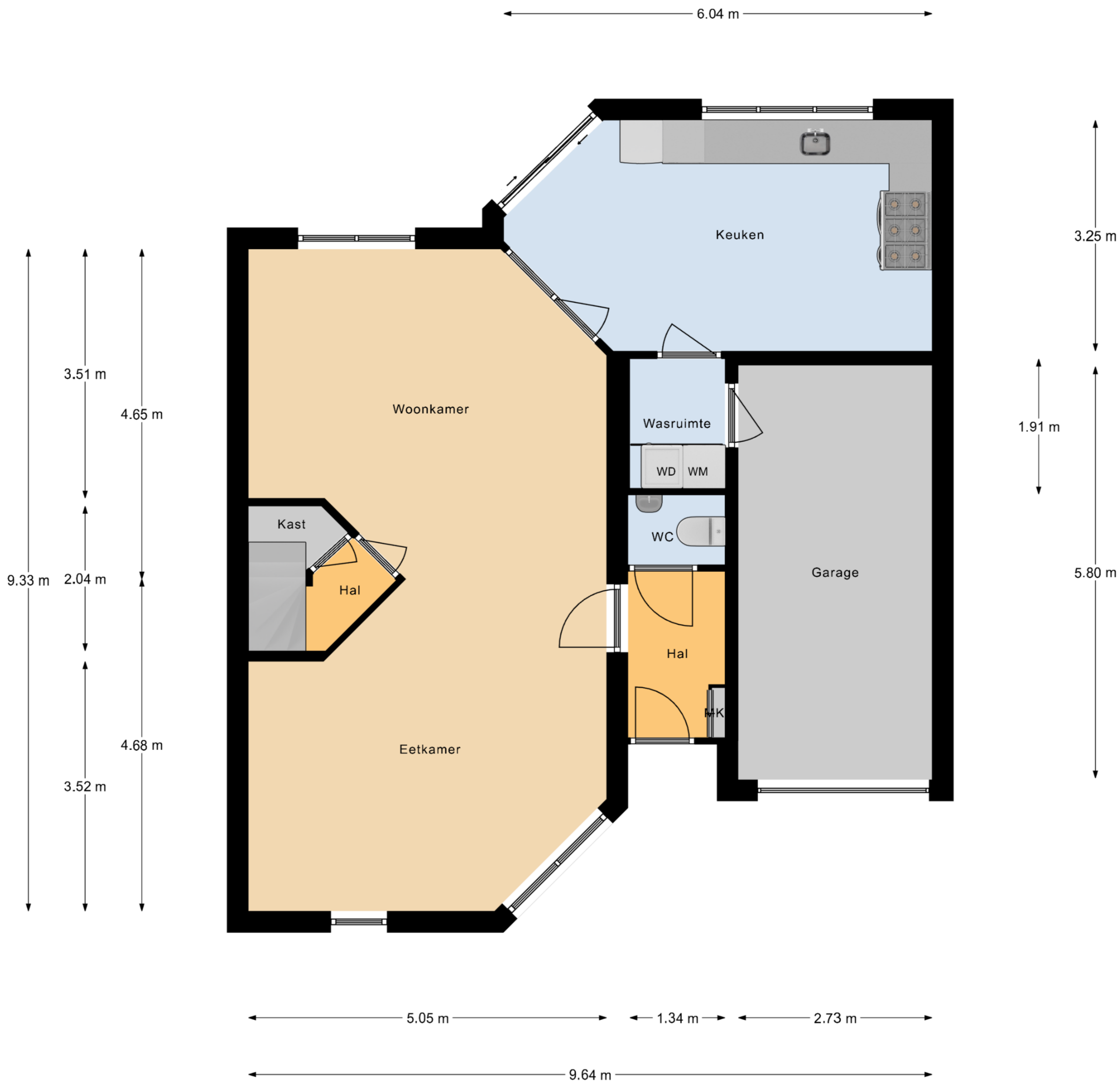
Begane Grond
