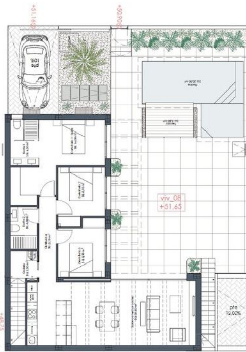
PLANTA BAJA
