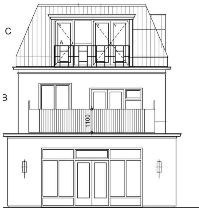
achter aanzicht
