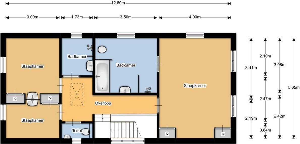
1e verdieping
