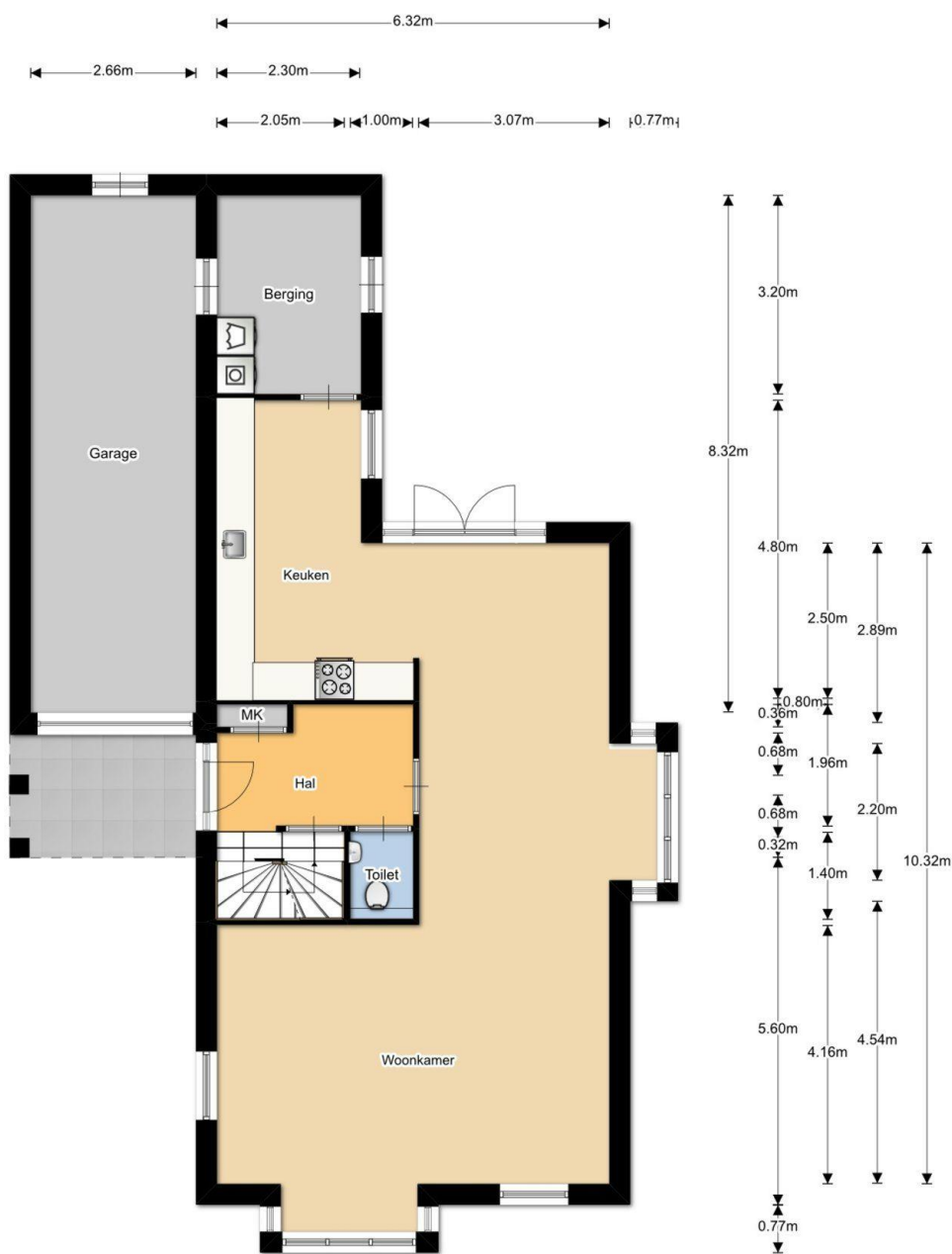
Begane grond
