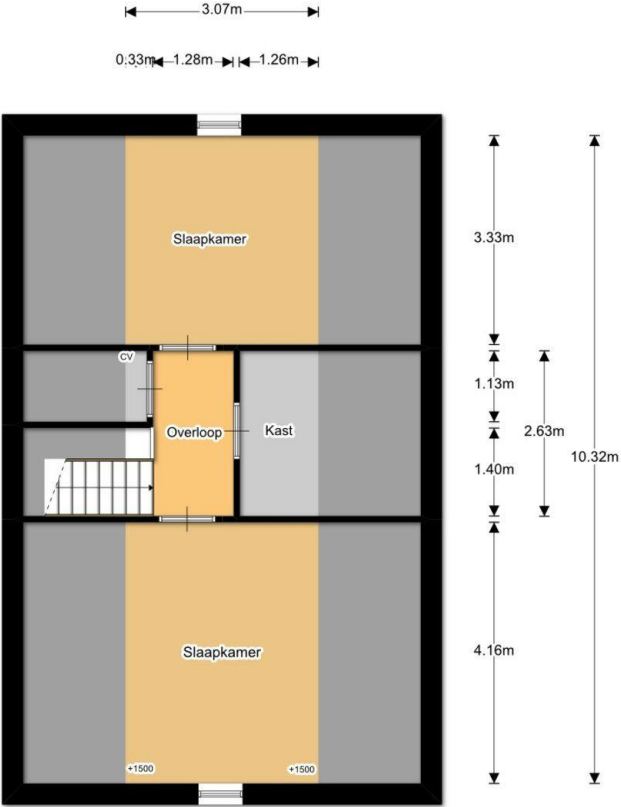
2e verdieping
