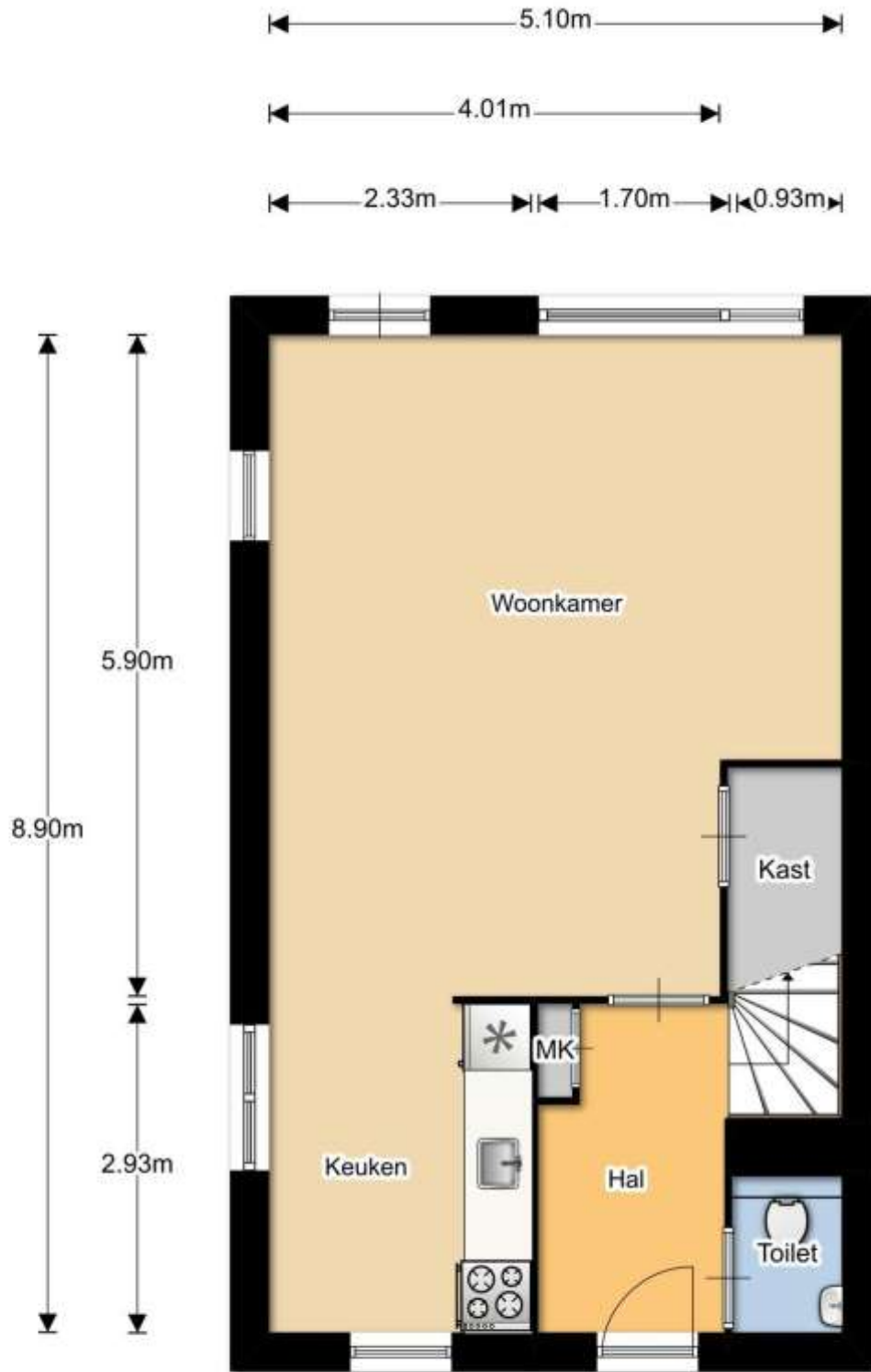
Begane grond
