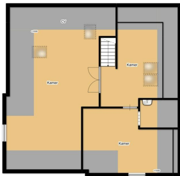
2e Verdieping
