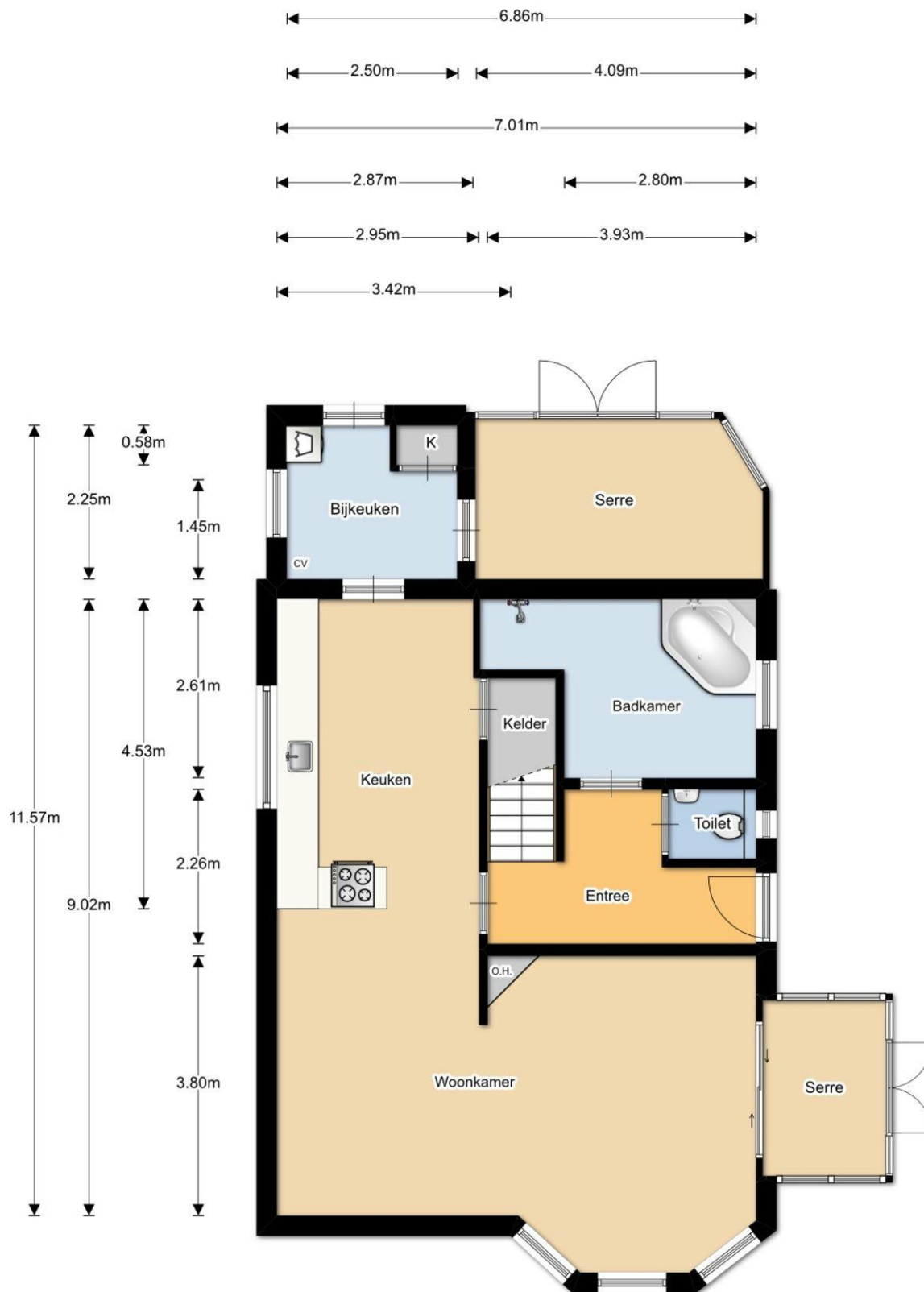
Begane grond
